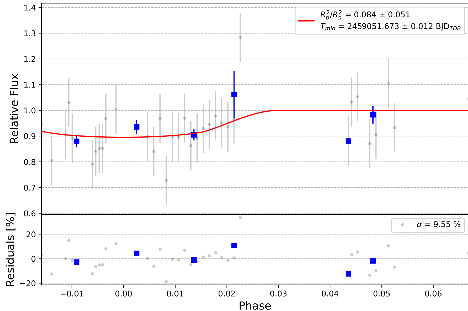
CoRoT-2 b
