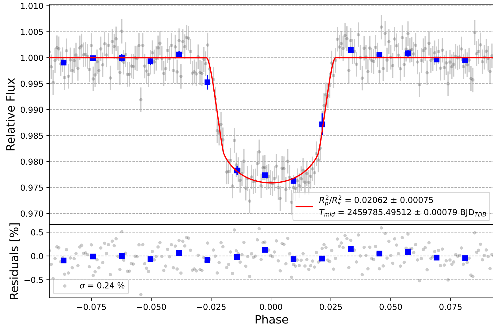
CoRoT-2 b
