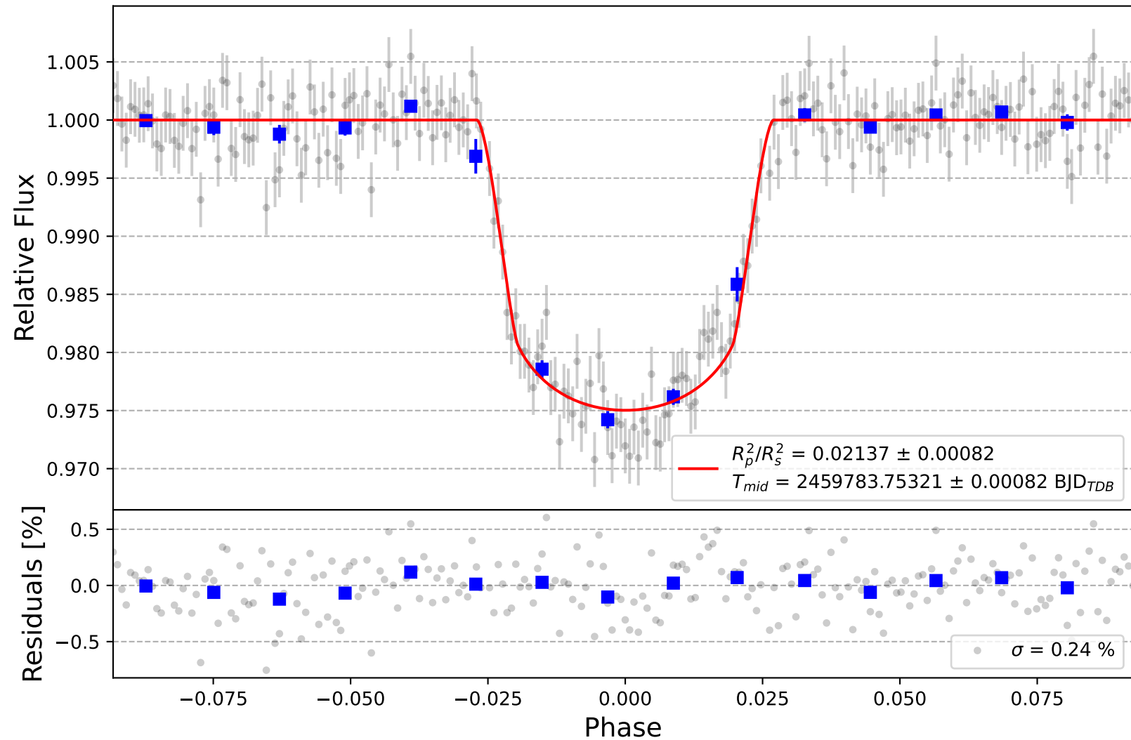
CoRoT-2 b
