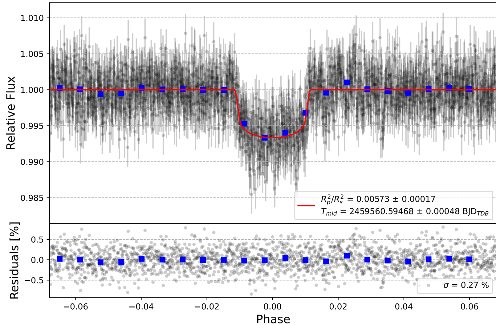
GJ 3470 b
