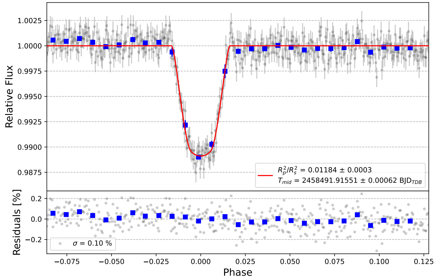
HAT-P-30 b
