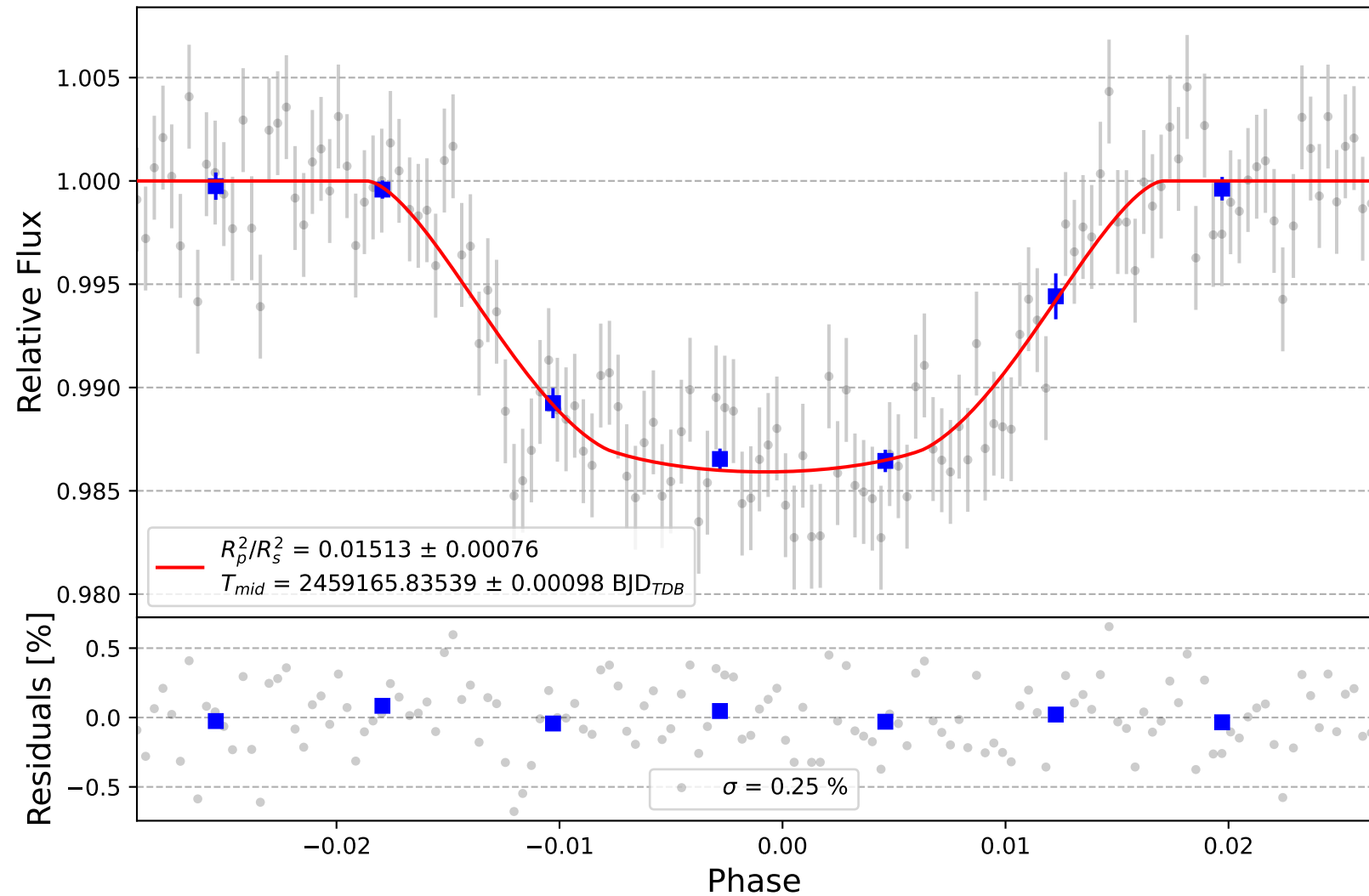
HAT-P-56 b
