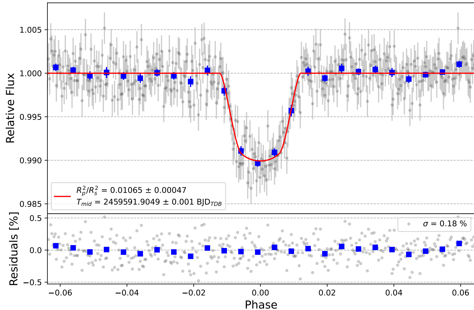
HAT-P-59 b
