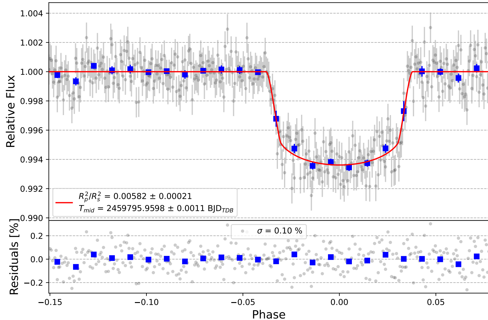
HAT-P-7 b
