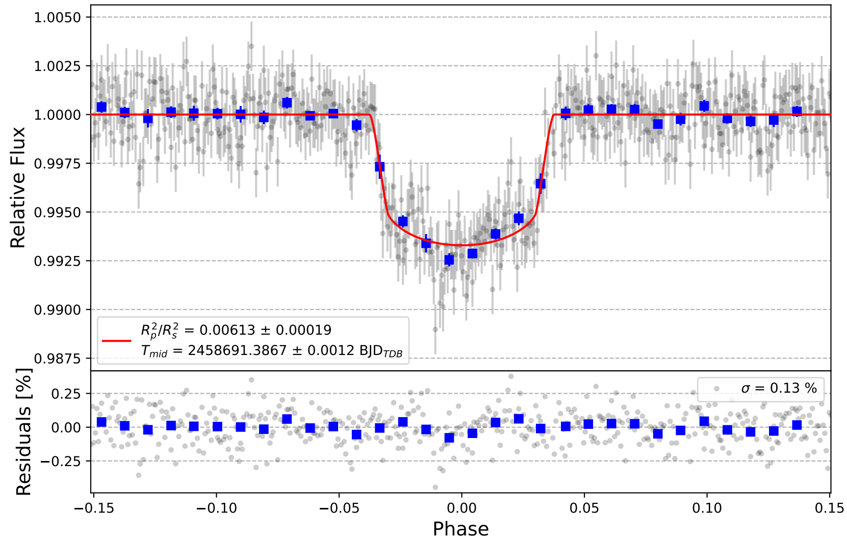
HAT-P-7 b
