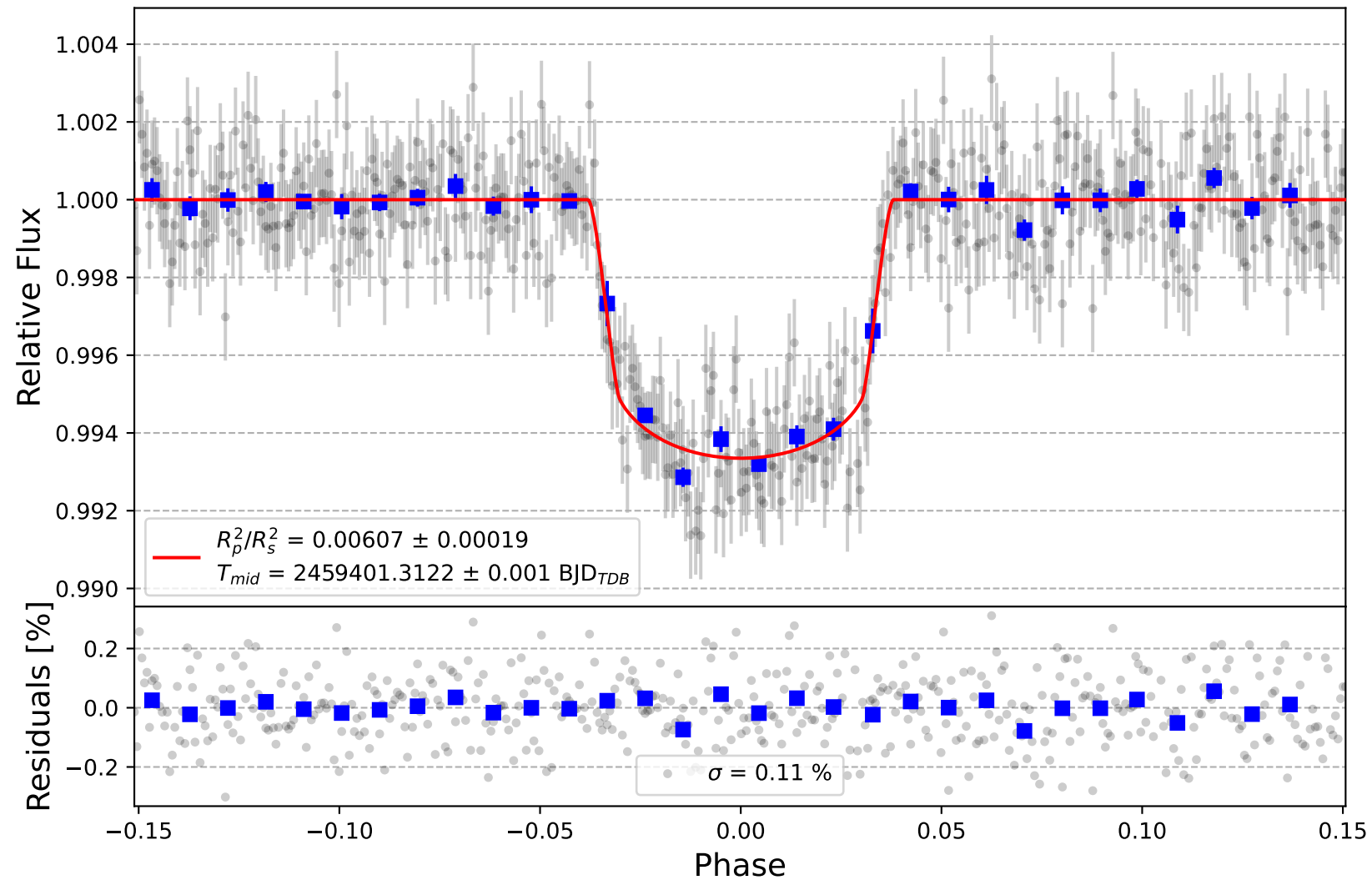
HAT-P-7 b
