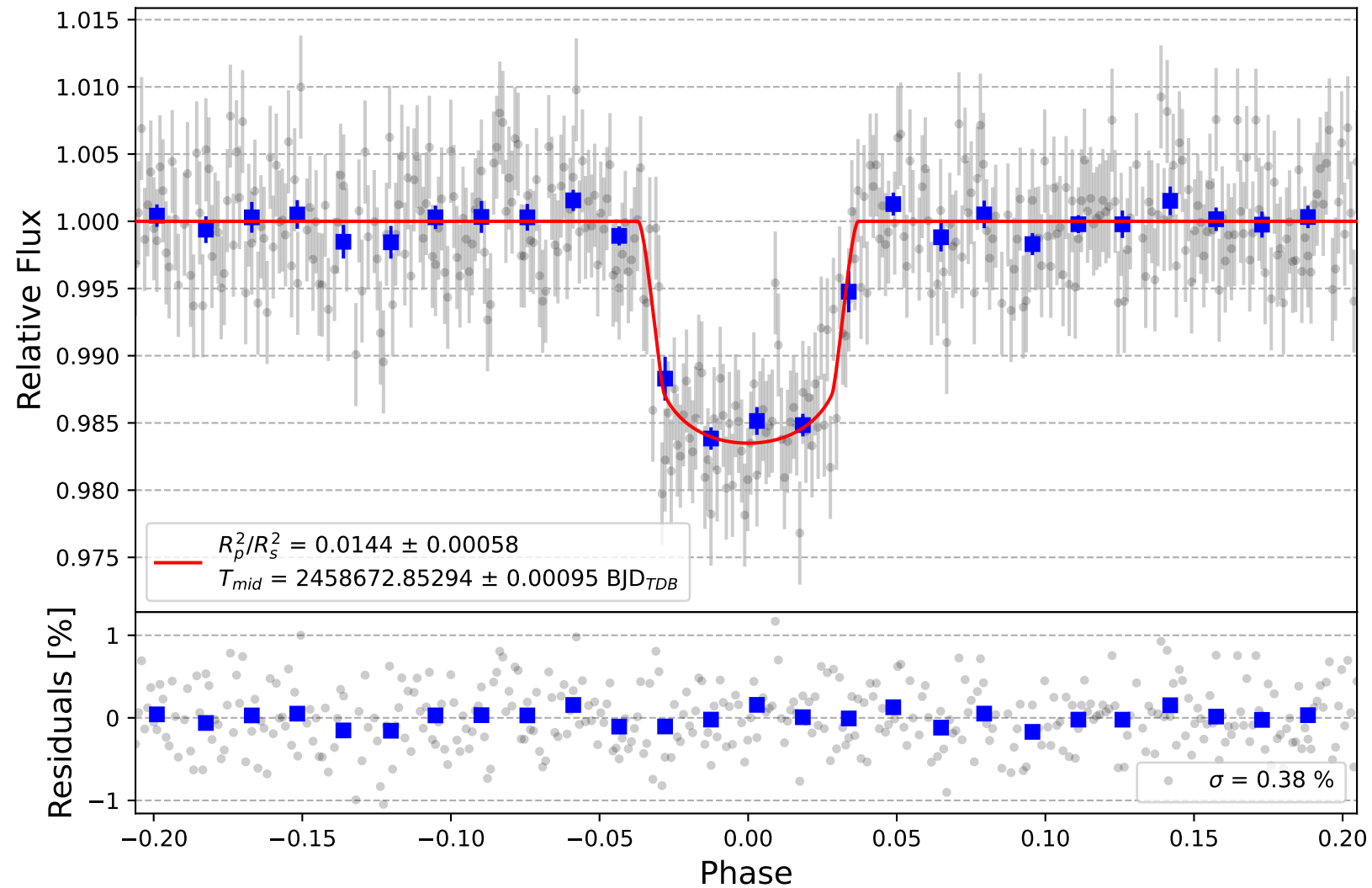
HATS-24 b
