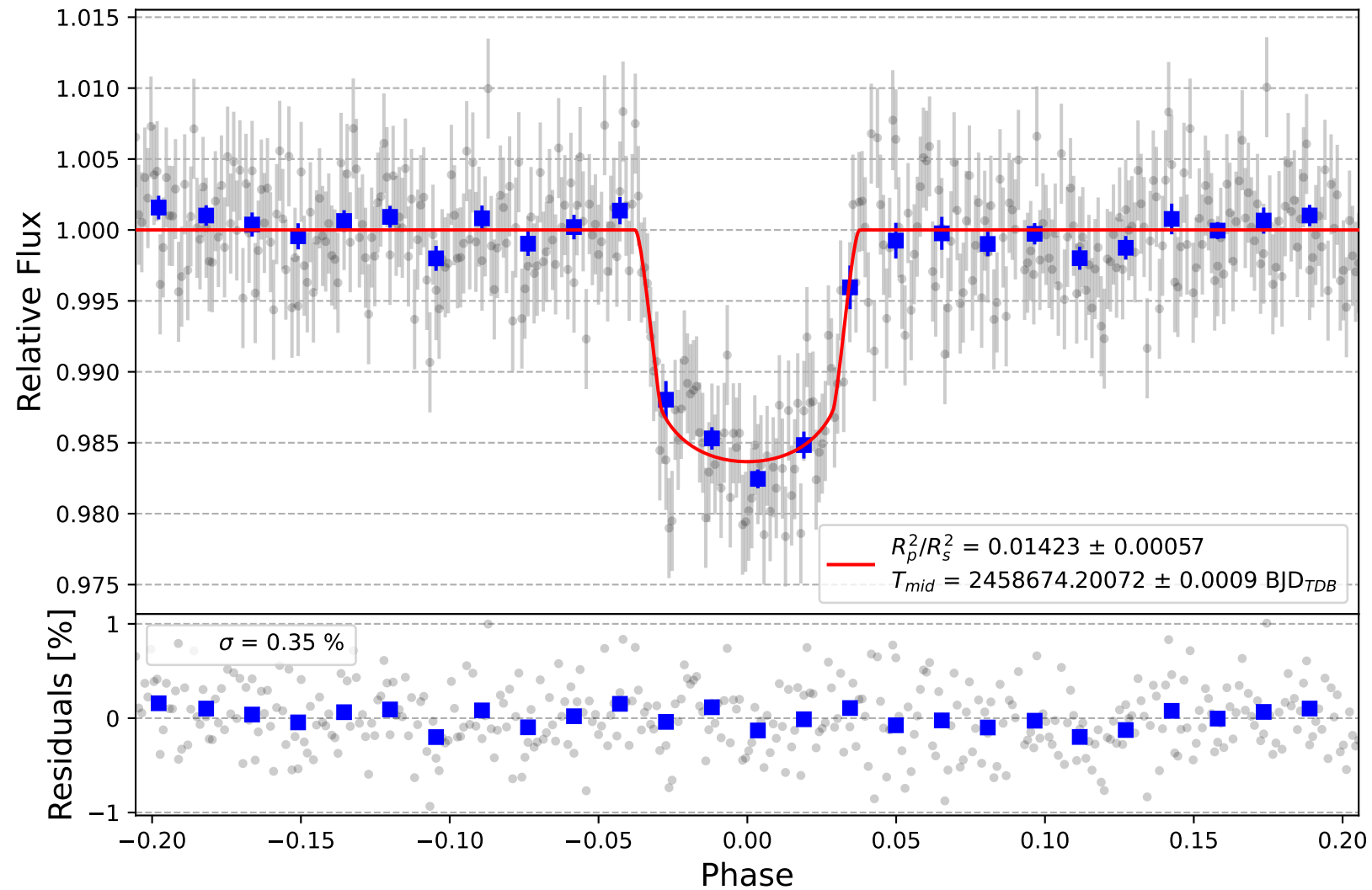
HATS-24 b
