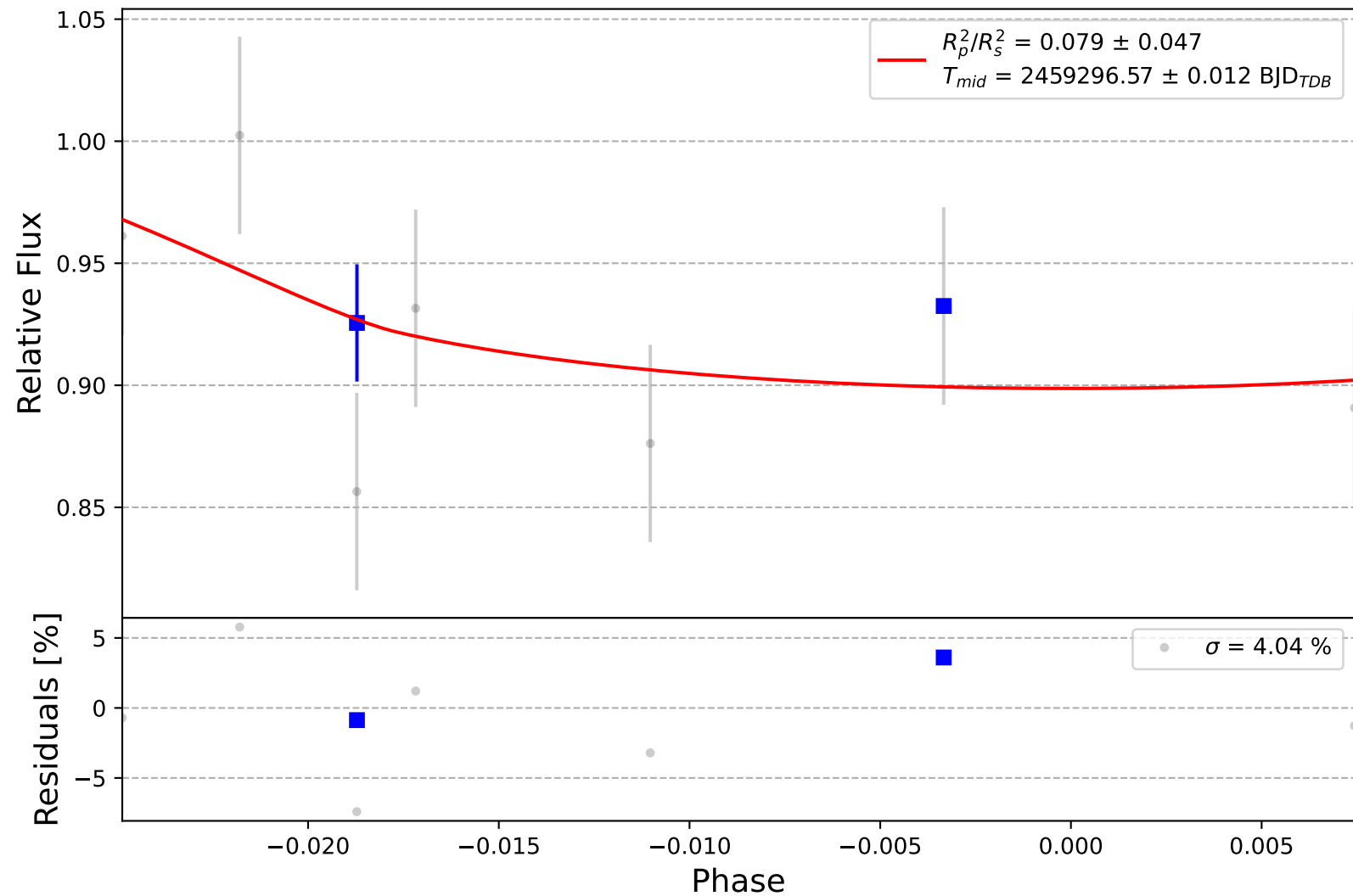
HATS-2 b
