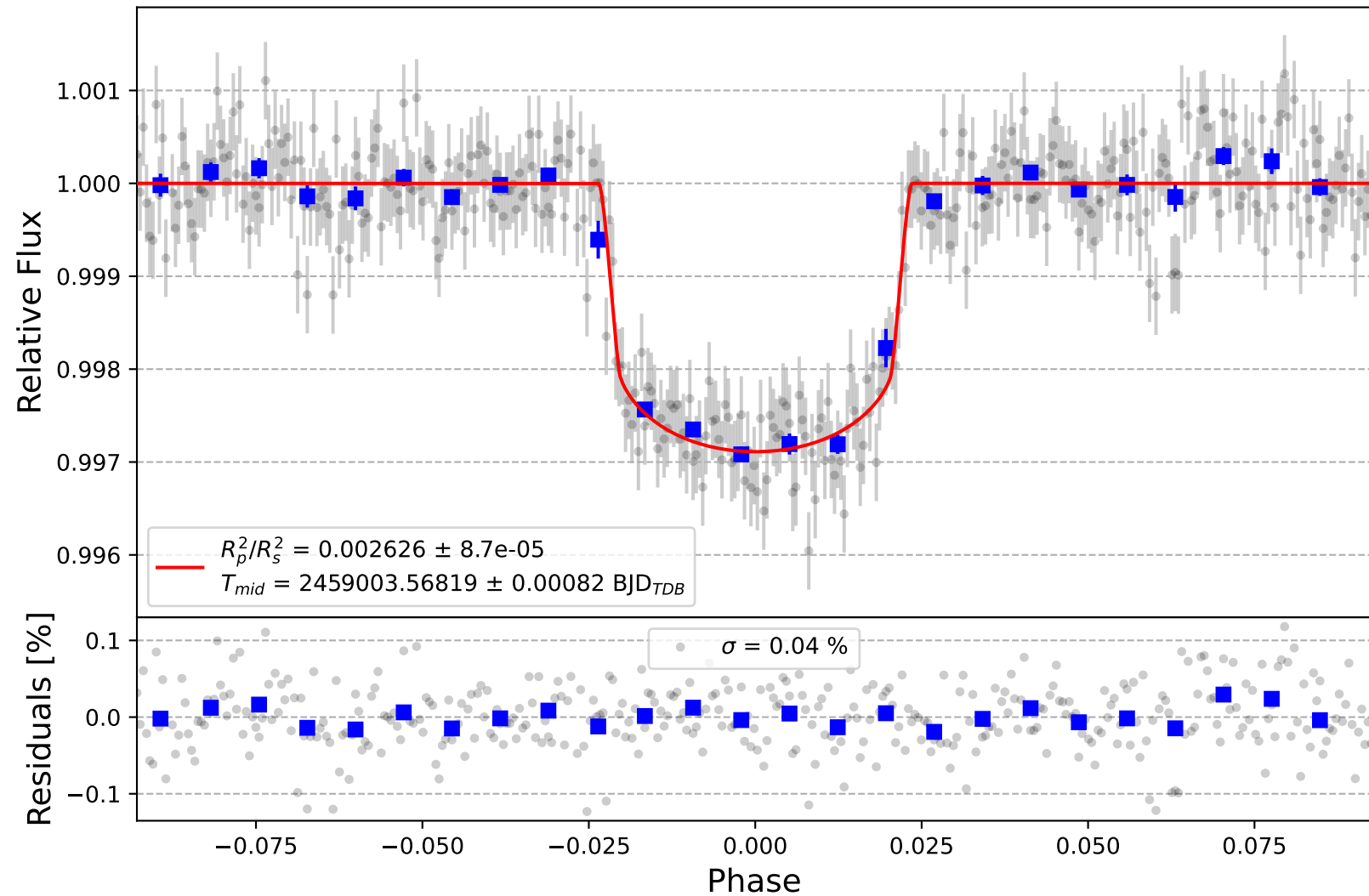
HD 149026 b
