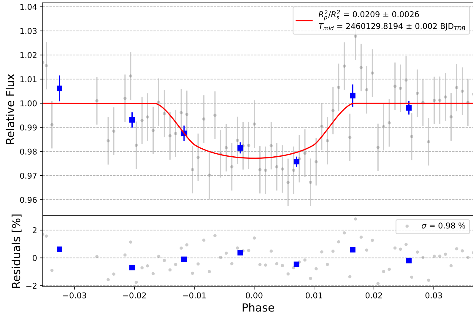
HD 189733 b
