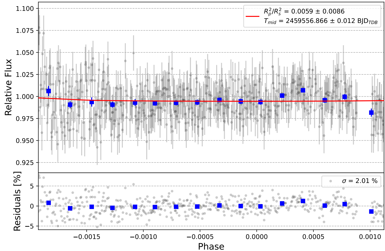
HD 80606 b
