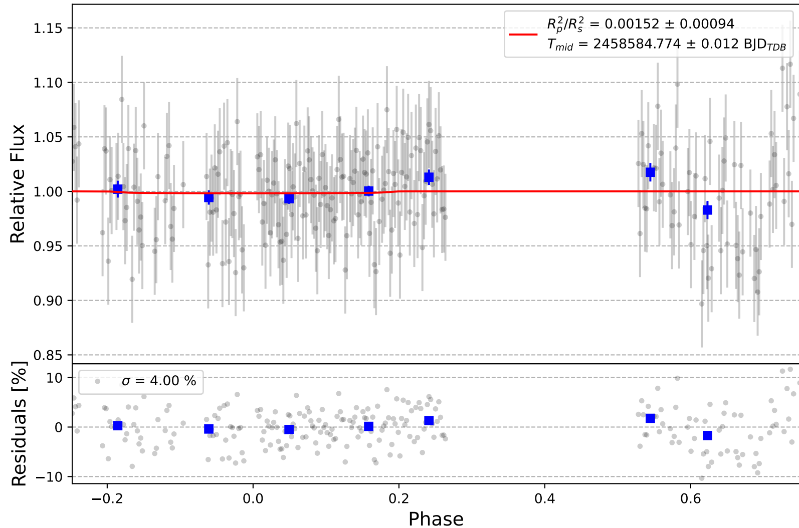
K2-137 b
