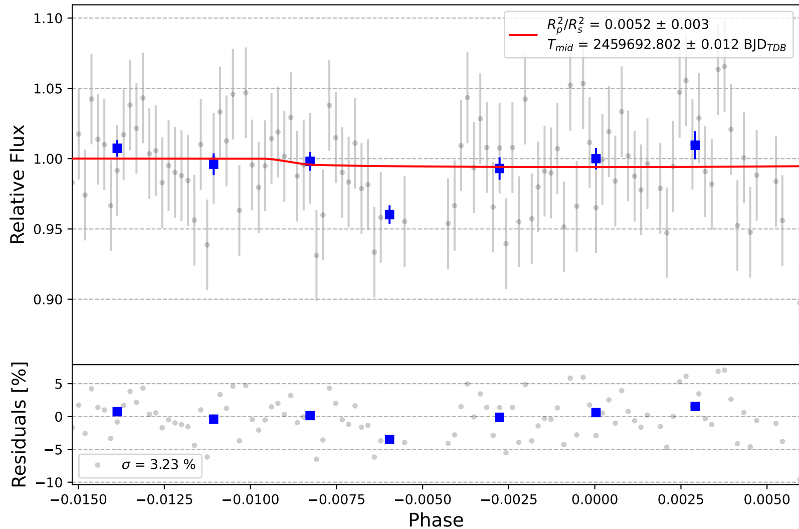
K2-153 b
