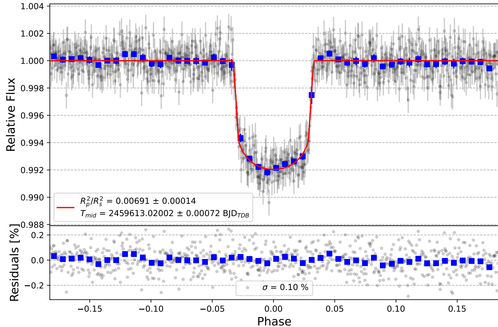
KELT-18 b
