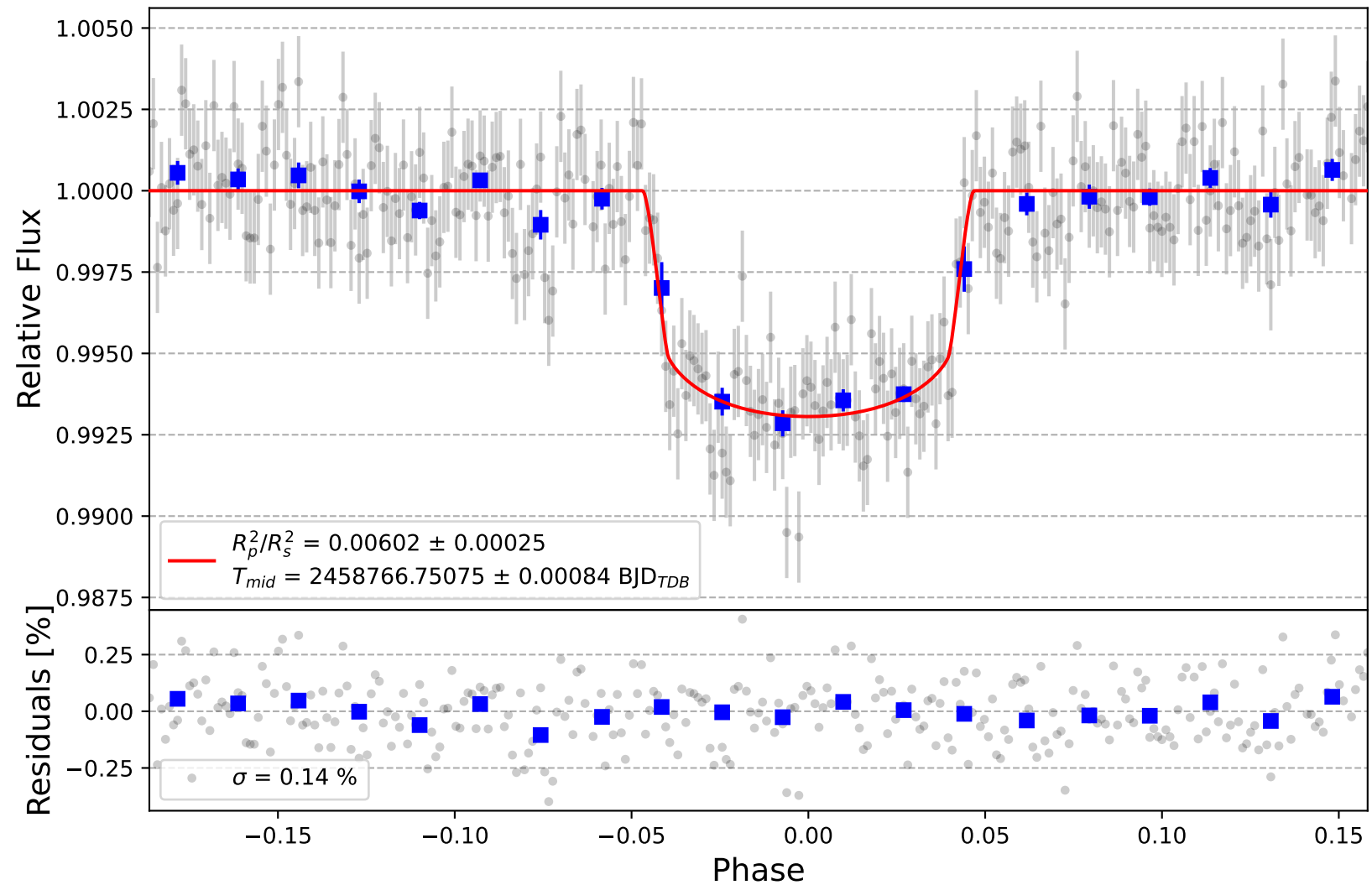
KELT-1 b
