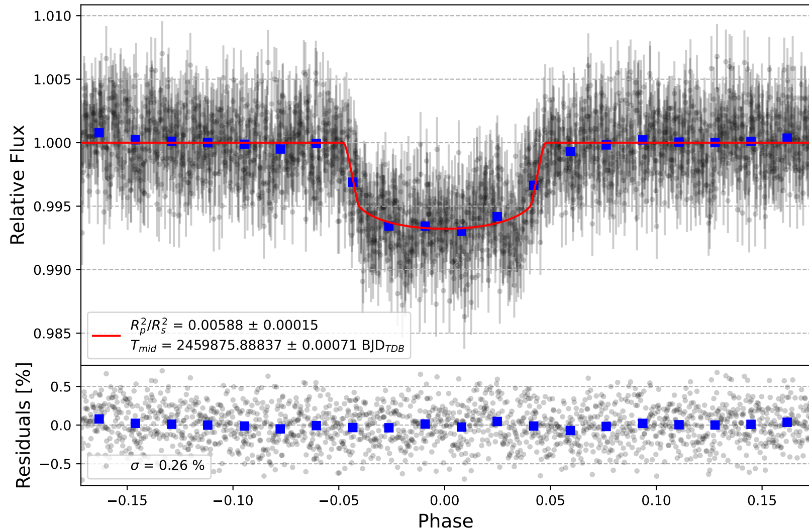
KELT-1 b
