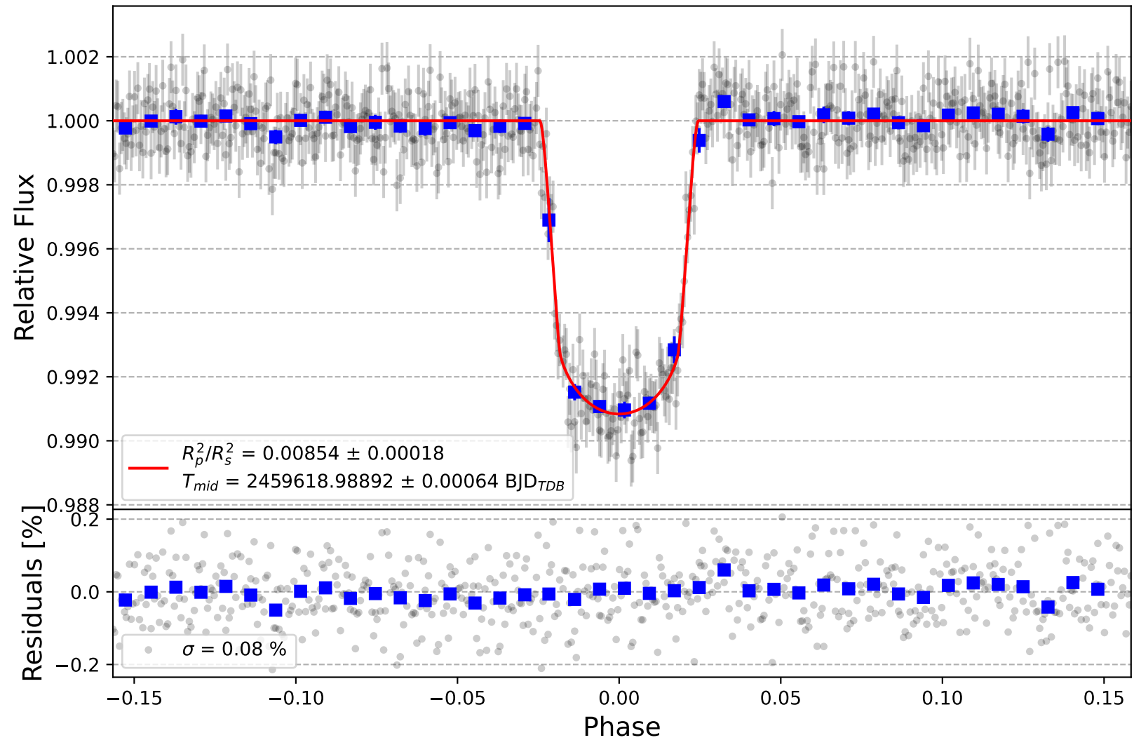
KELT-3 b
