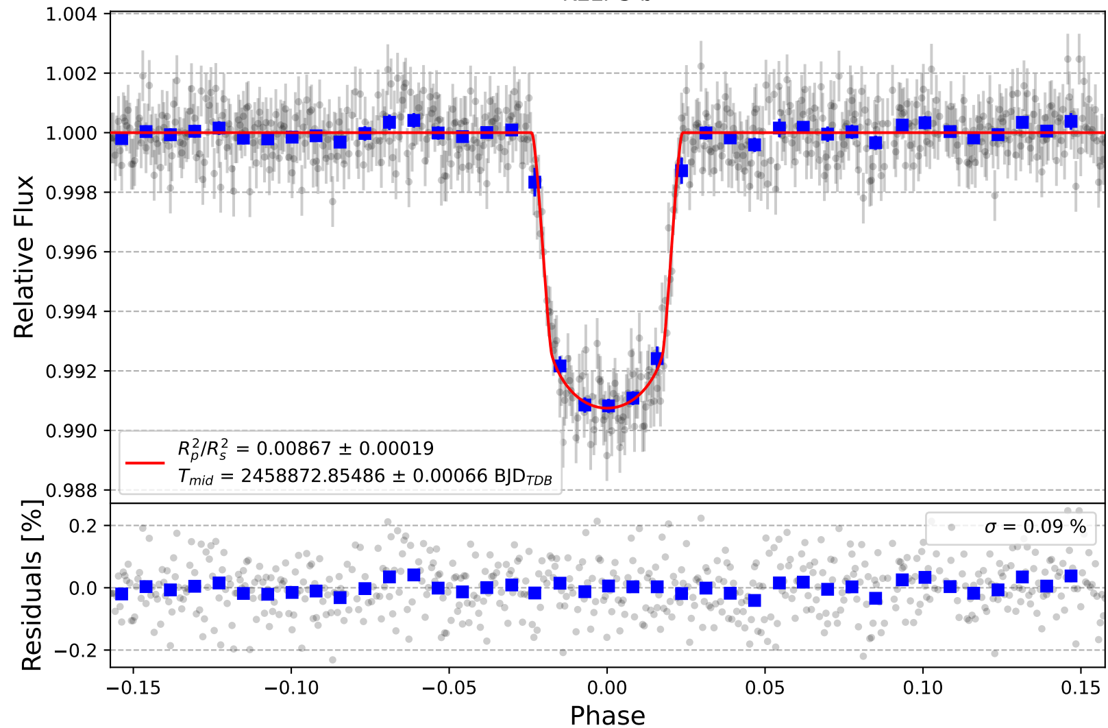
KELT-3 b
