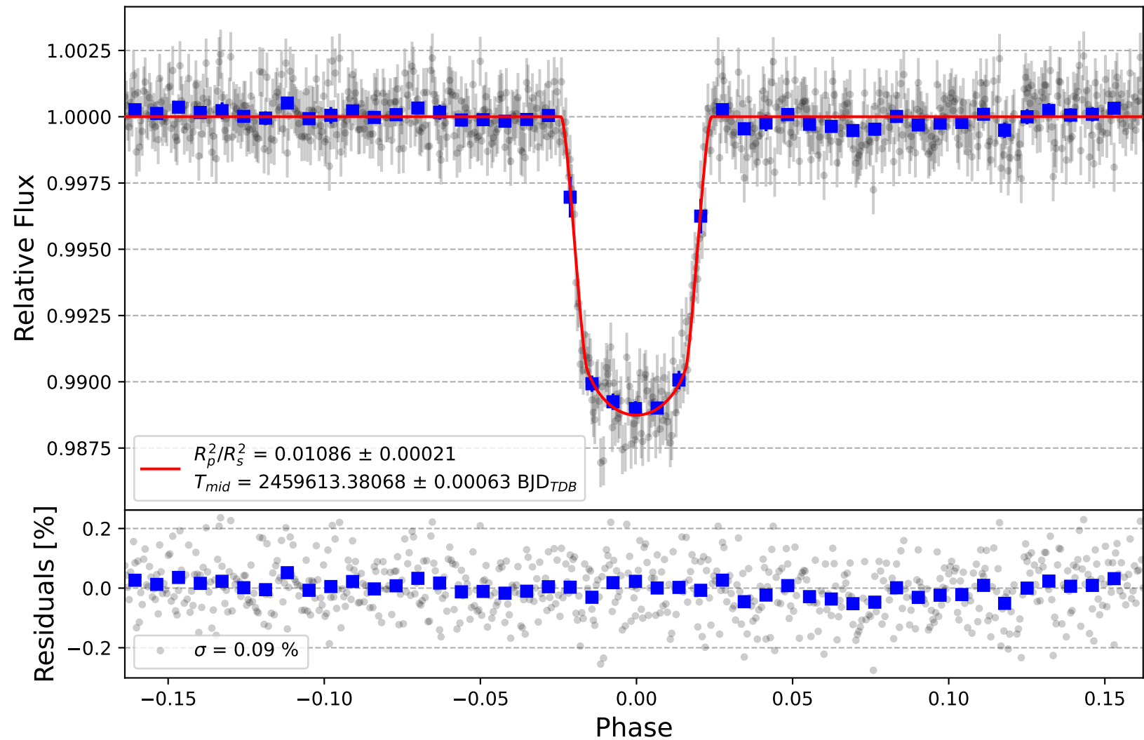
KELT-4 A b
