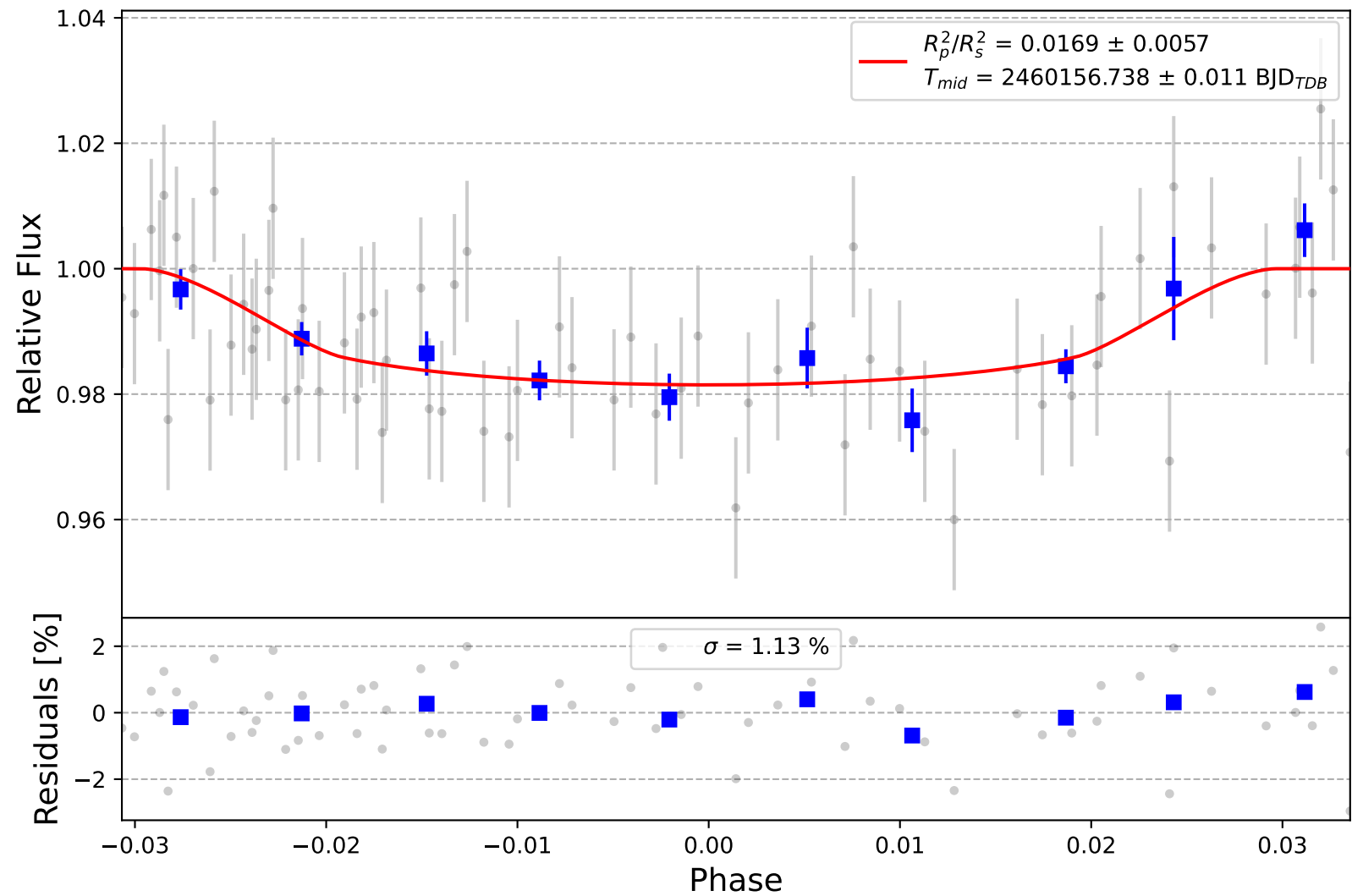
KELT-8 b
