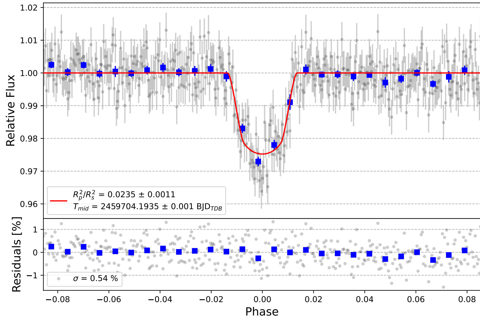
NGTS-5 b
