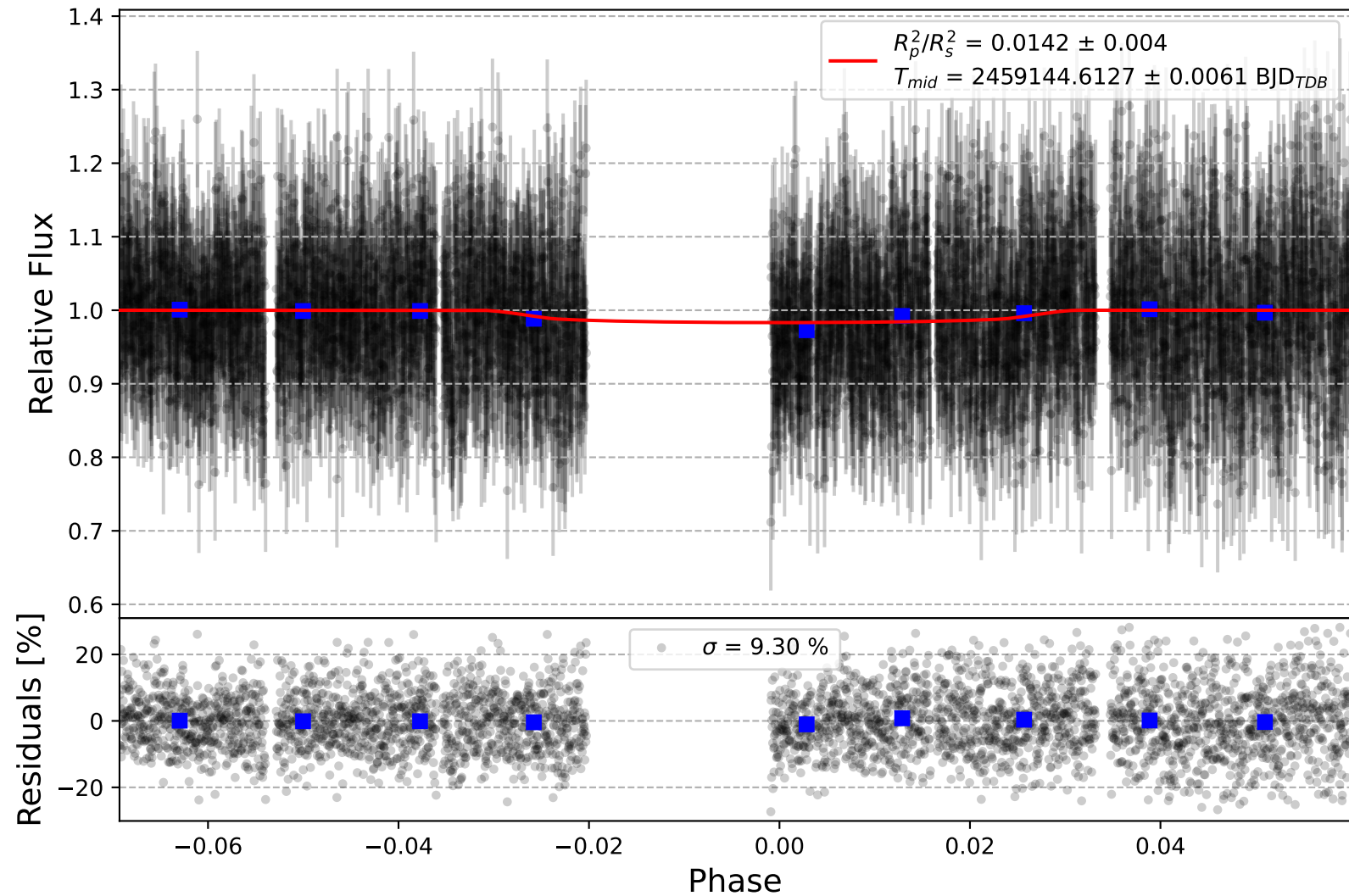
Qatar-10 b
