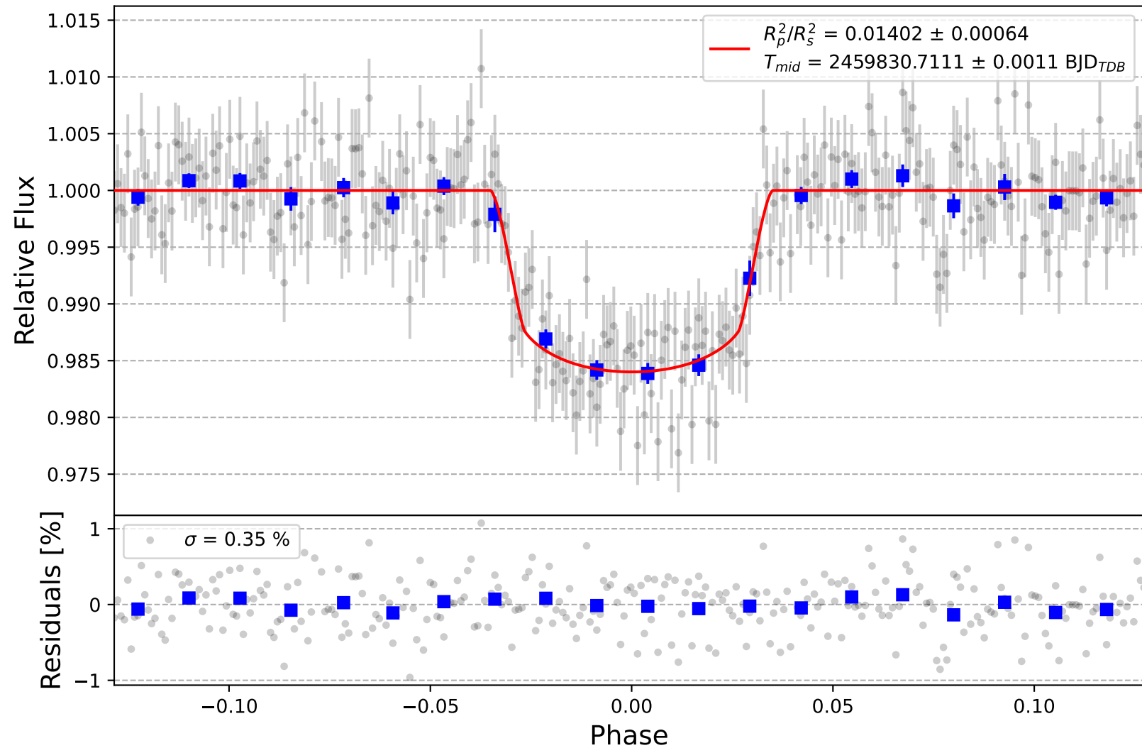
Qatar-10 b
