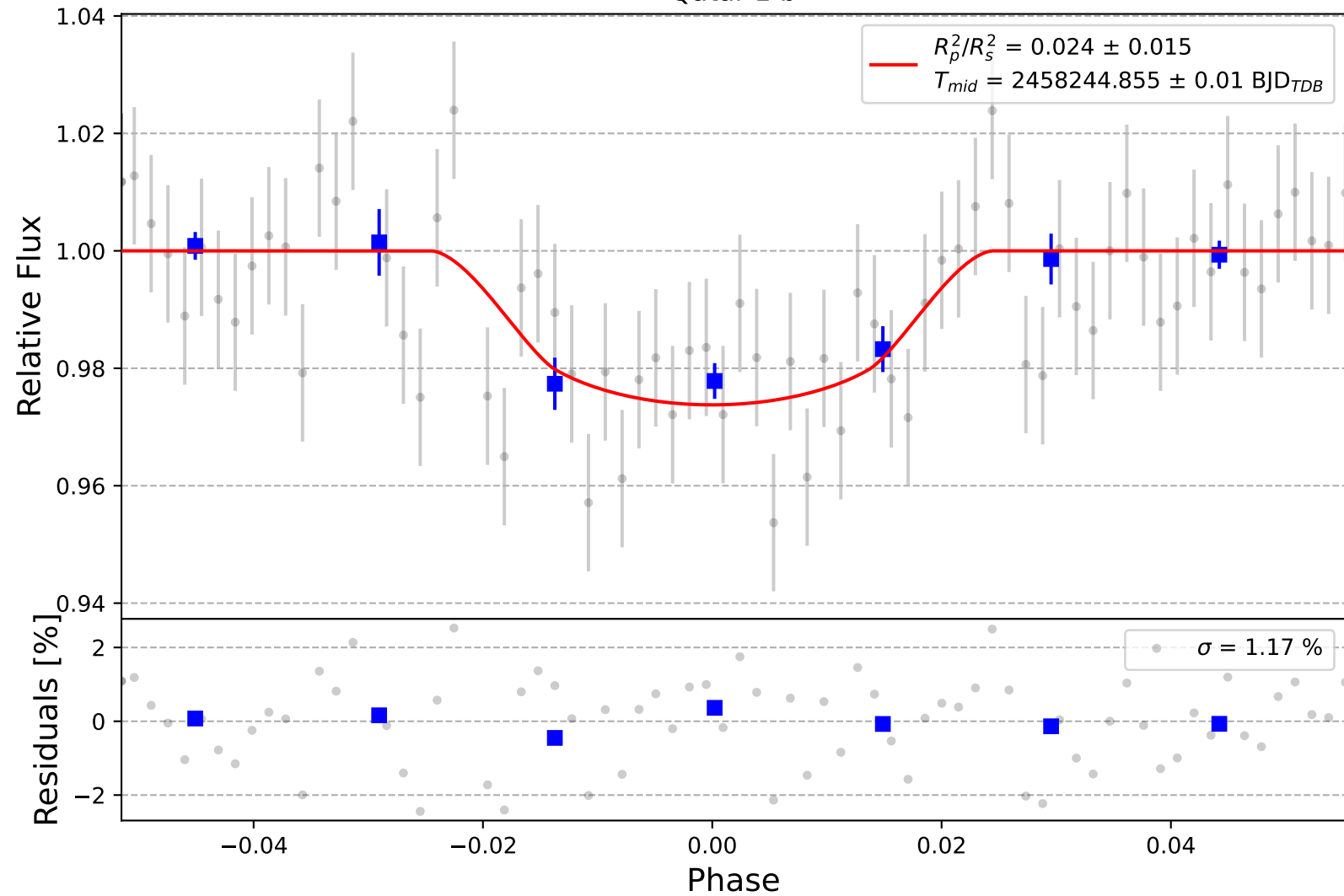
Qatar-1 b
