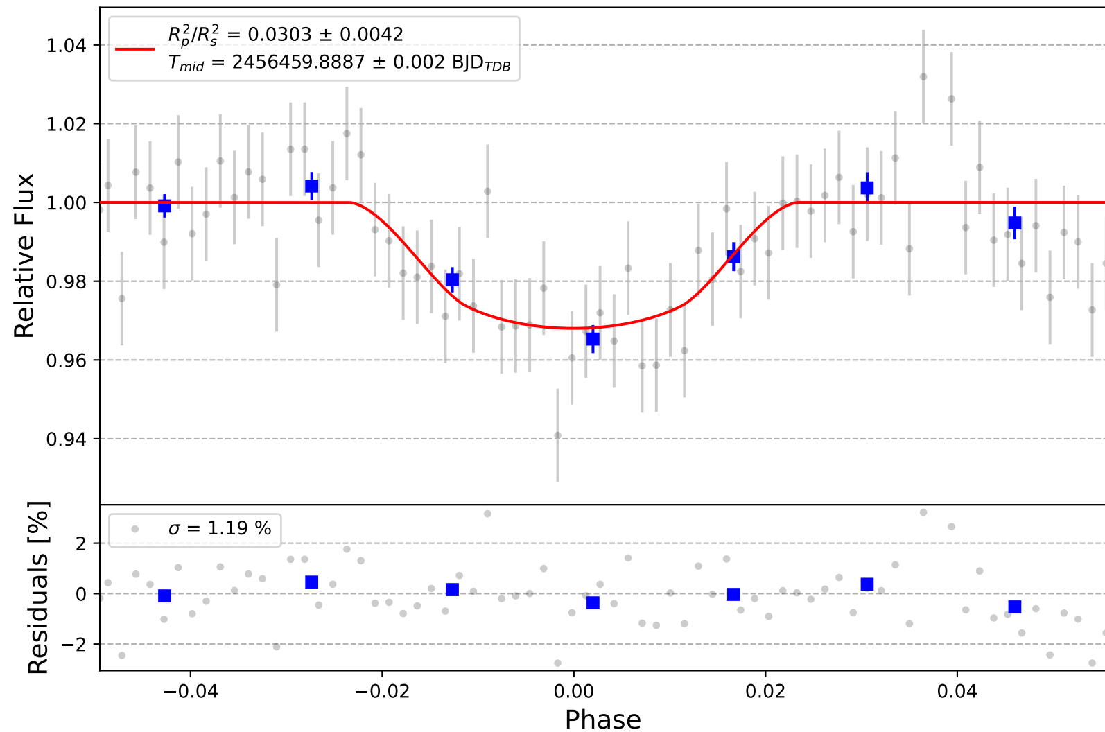
Qatar-1 b
