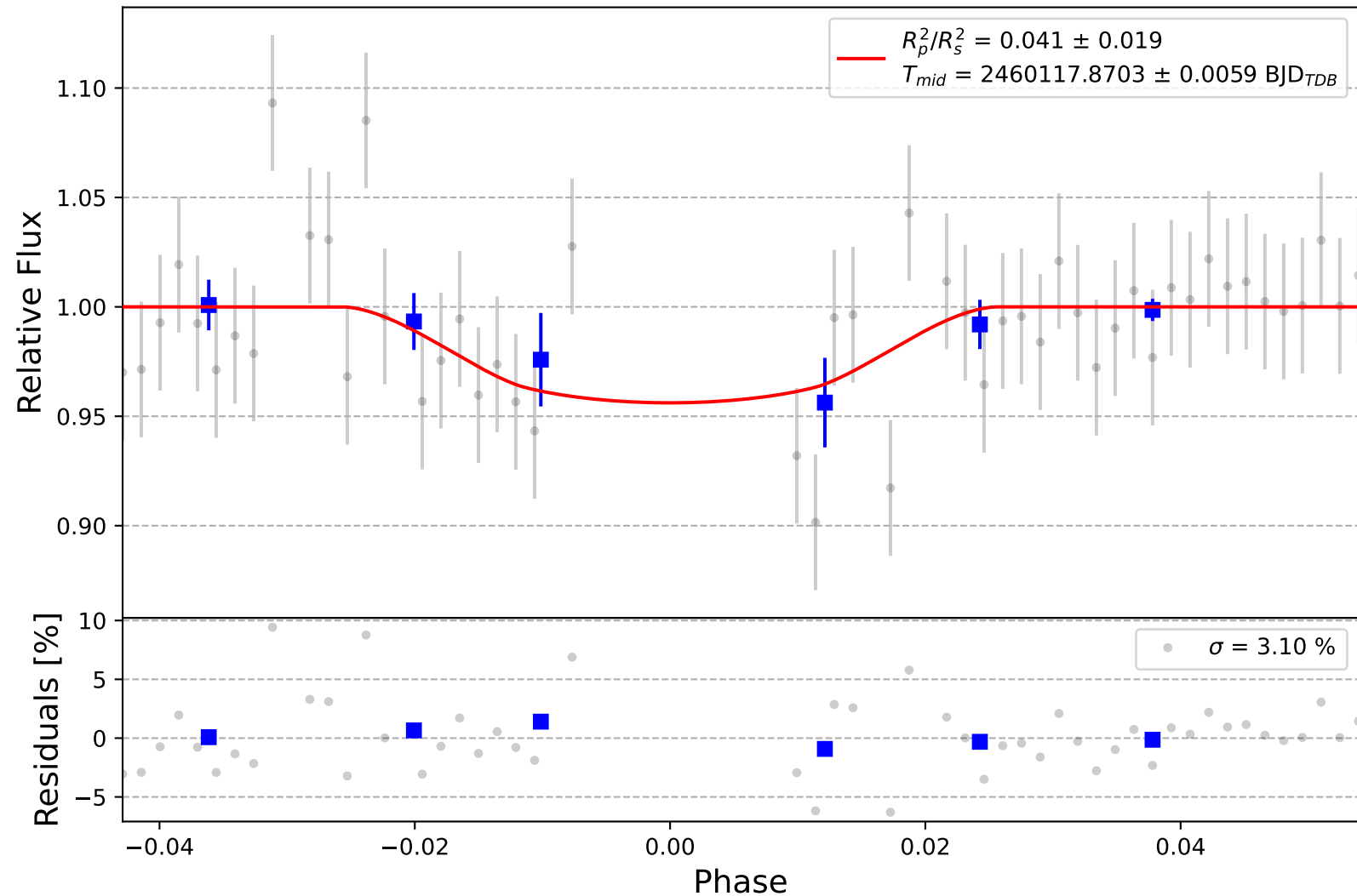
Qatar-1 b
