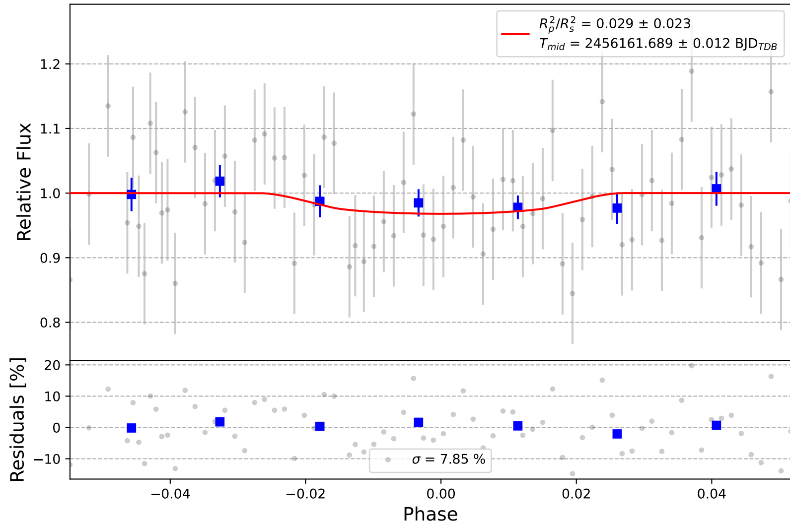
Qatar-1 b
