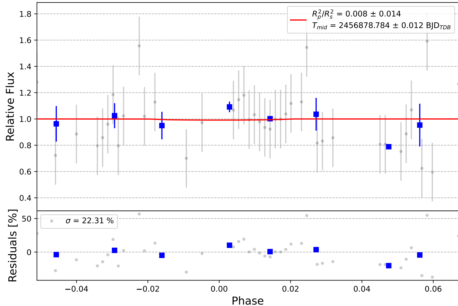
Qatar-1 b
