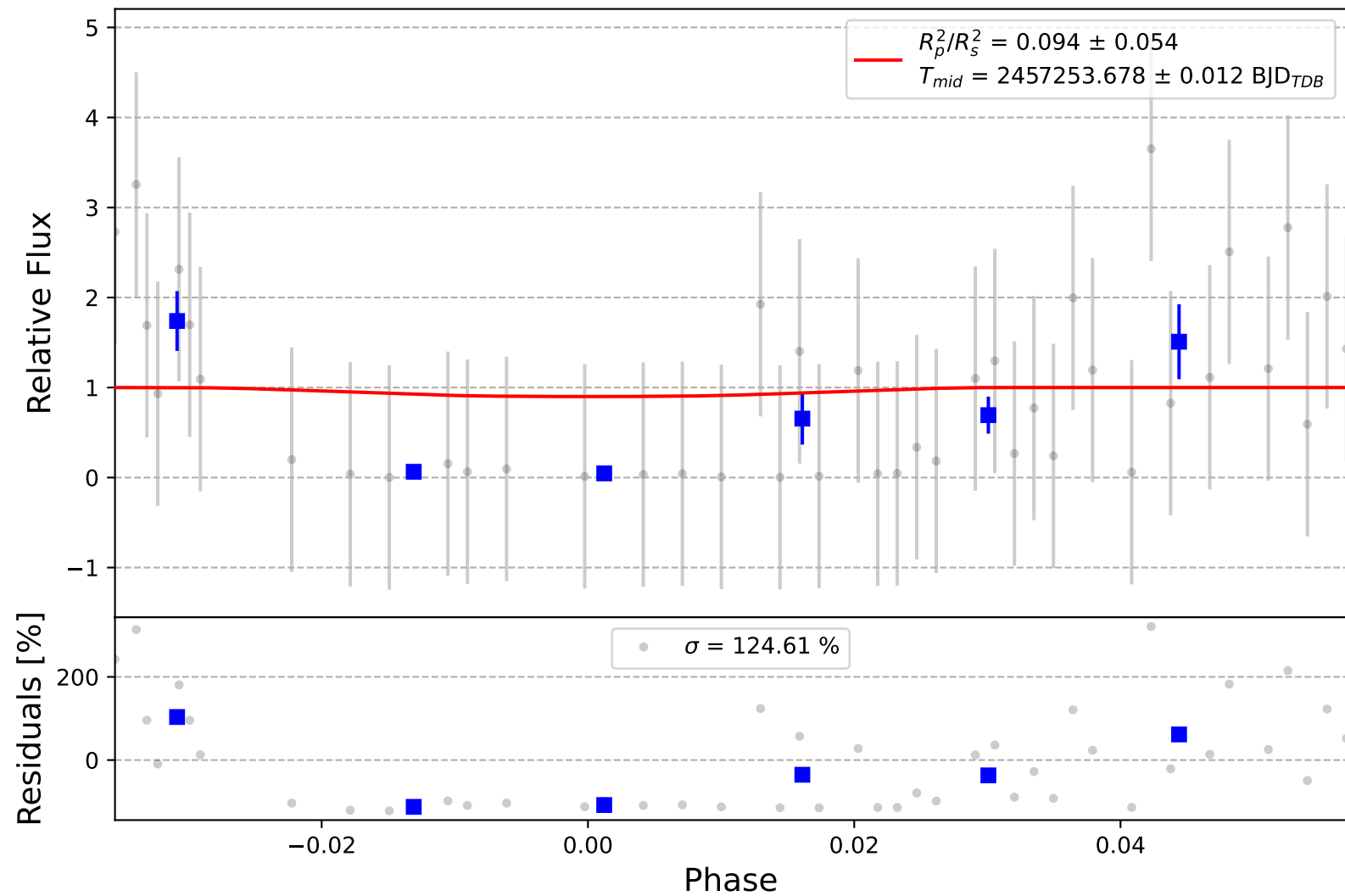
Qatar-1 b
