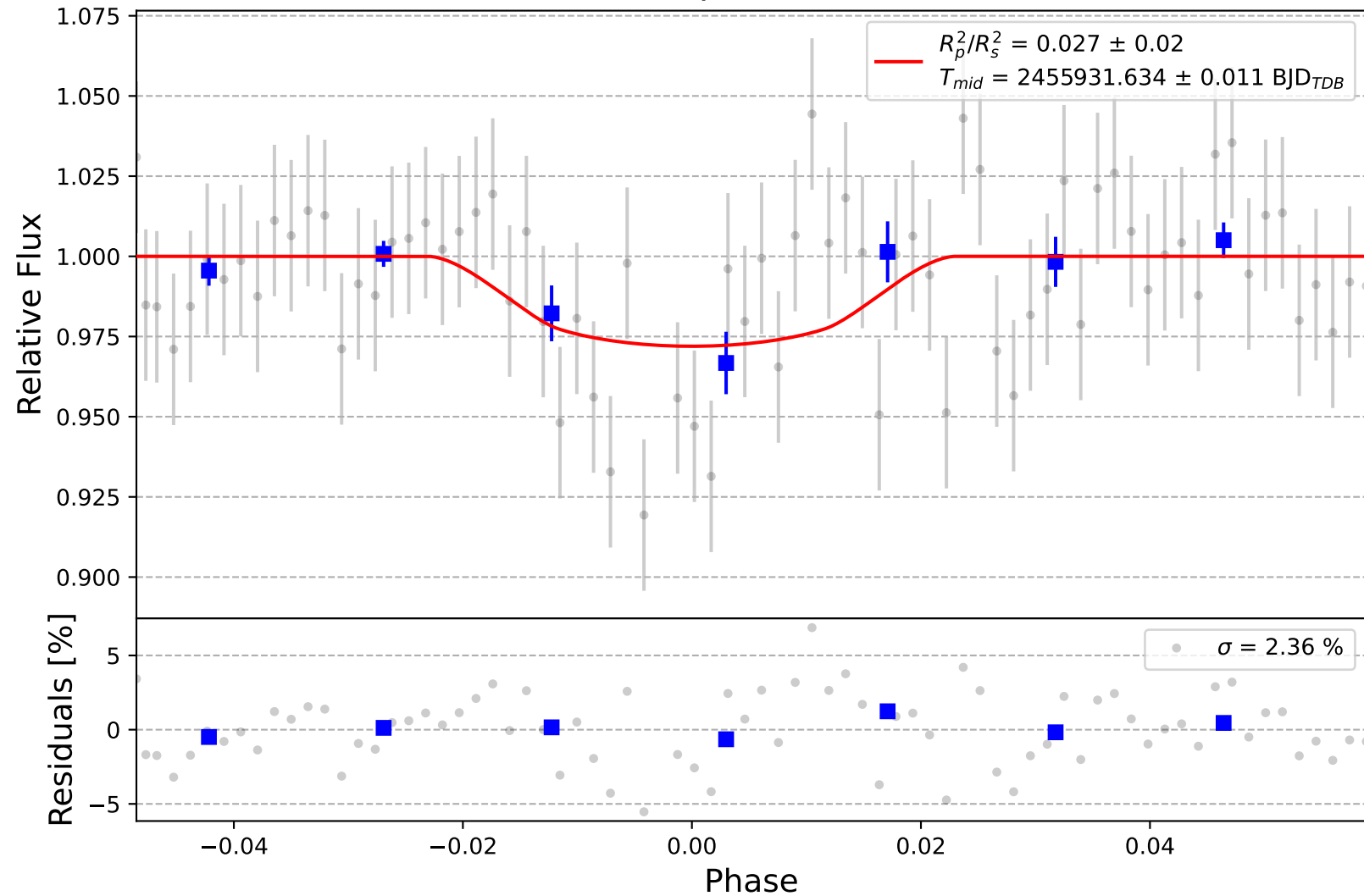
Qatar-1 b
