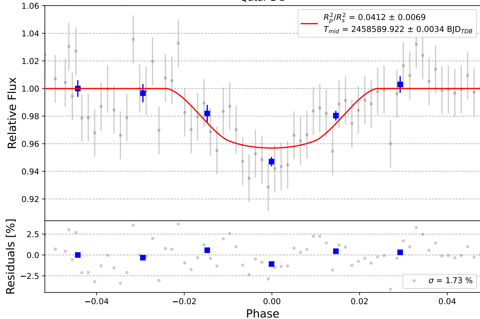
Qatar-1 b
