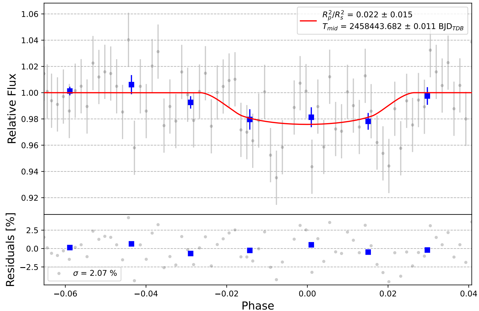
Qatar-1 b
