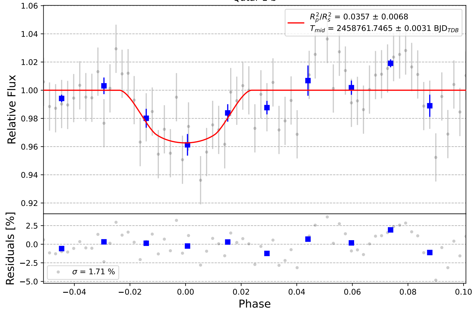
Qatar-1 b
