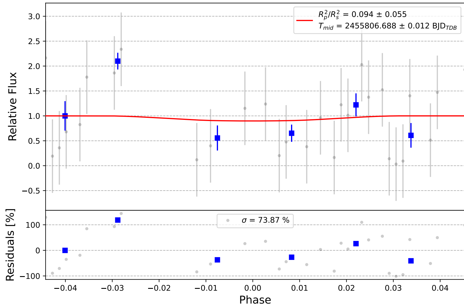
Qatar-1 b
