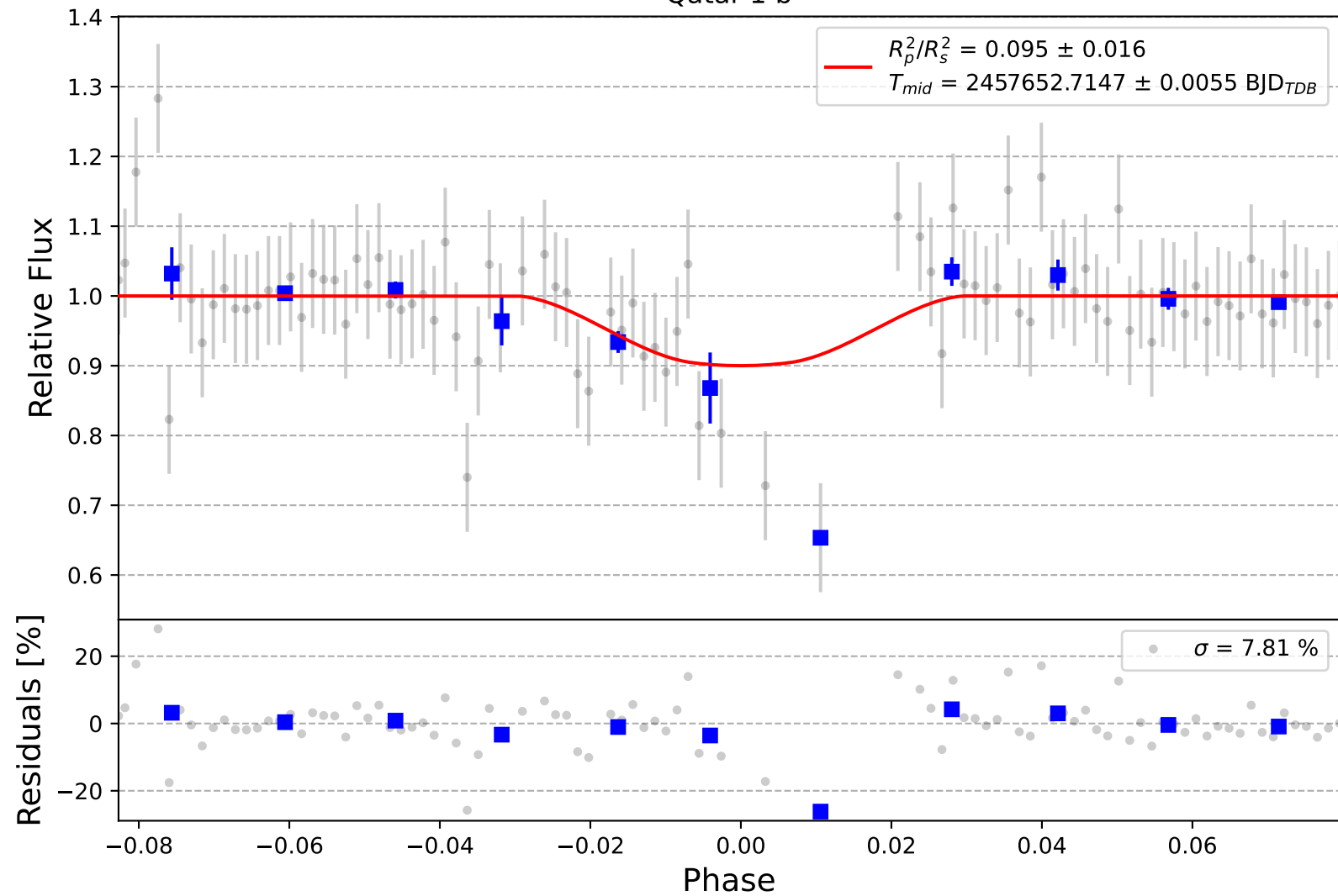
Qatar-1 b
