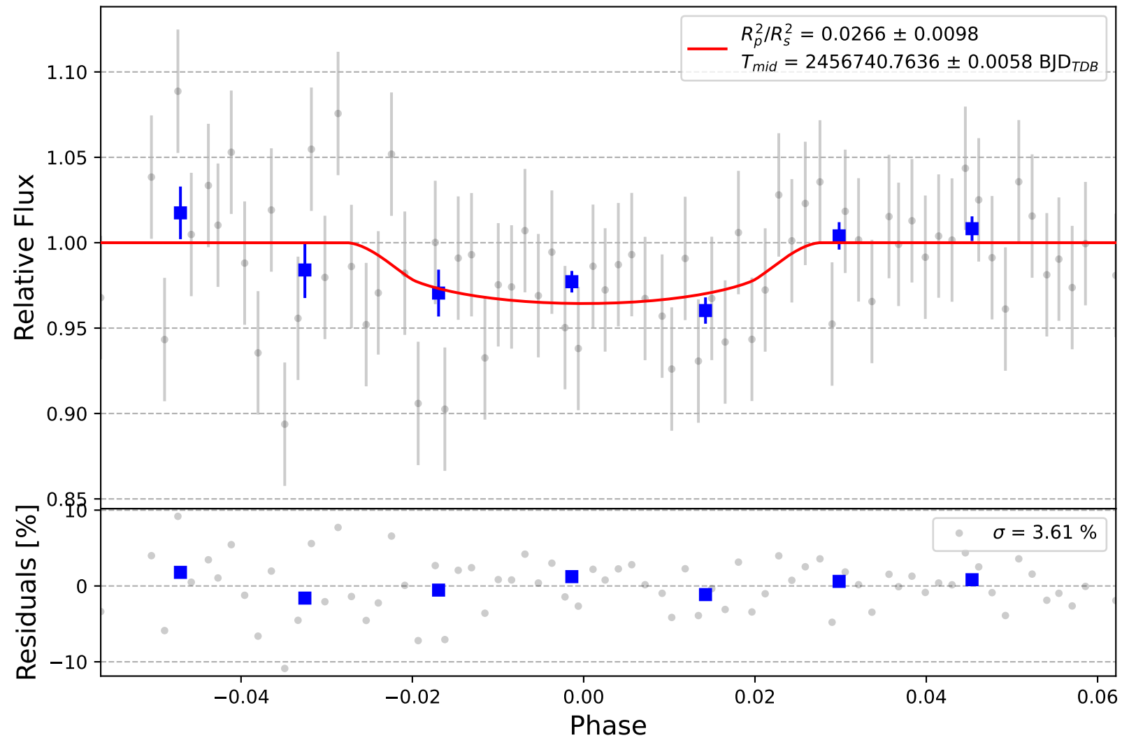
Qatar-2 b
