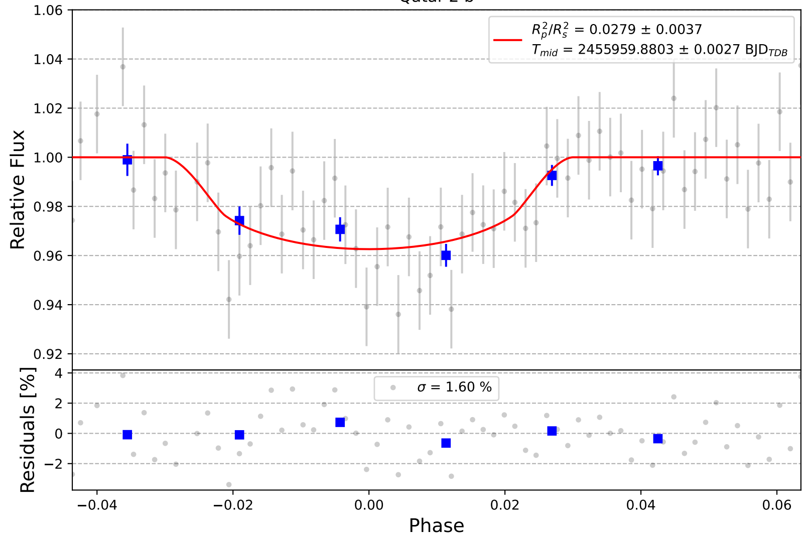
Qatar-2 b
