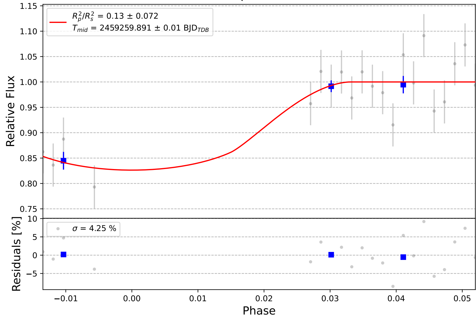
Qatar-2 b
