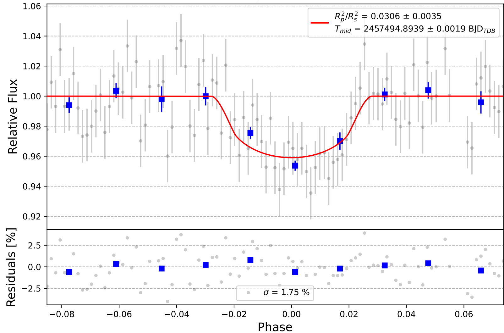
Qatar-2 b
