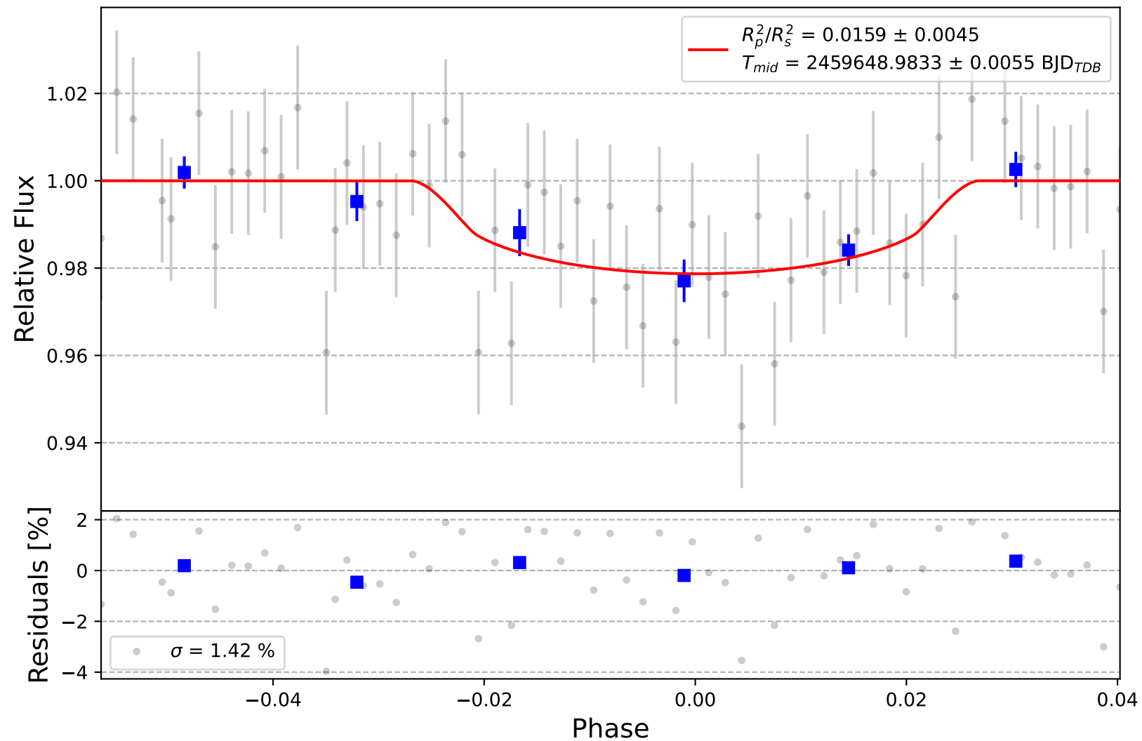
Qatar-2 b
