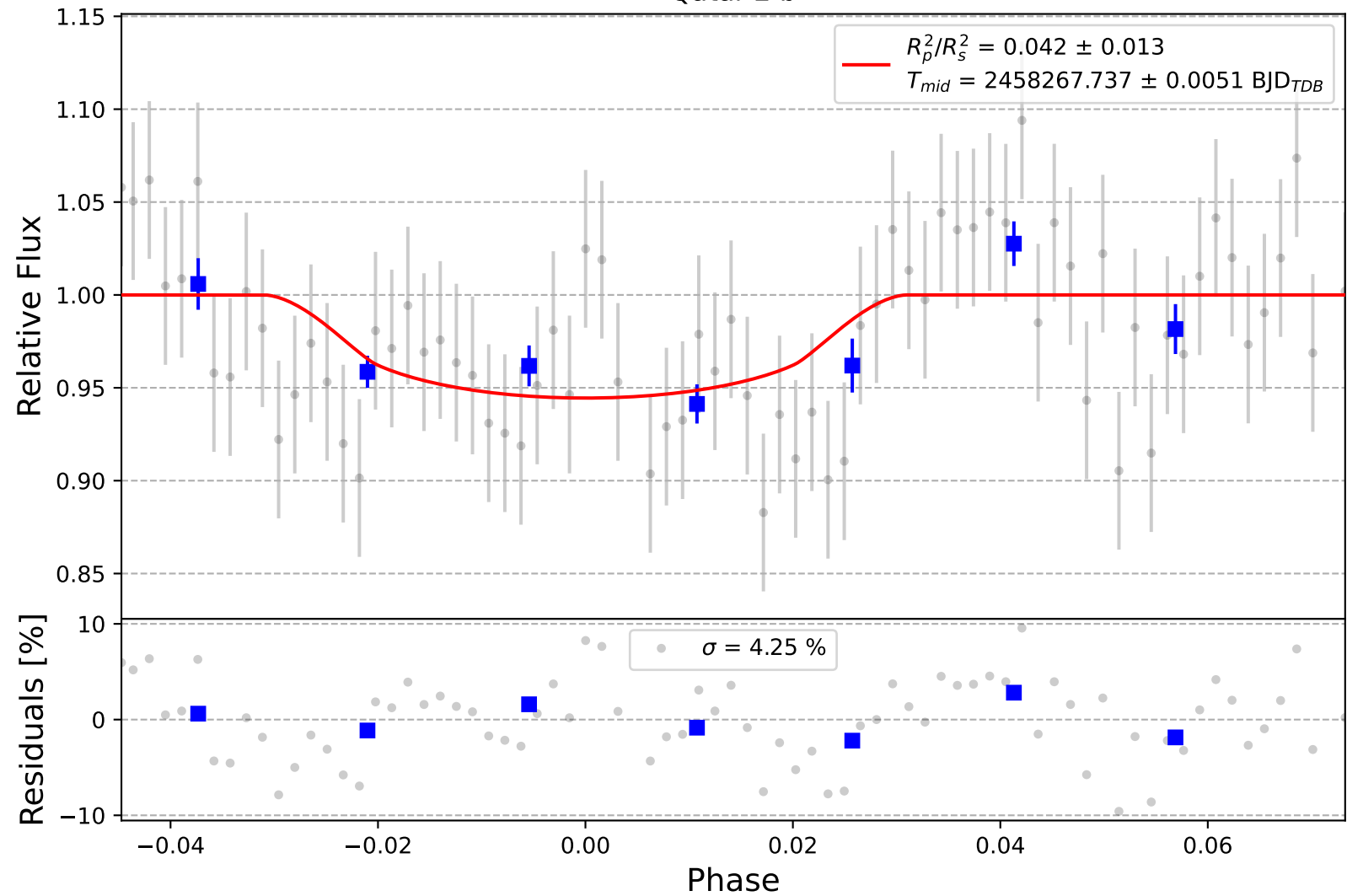
Qatar-2 b
