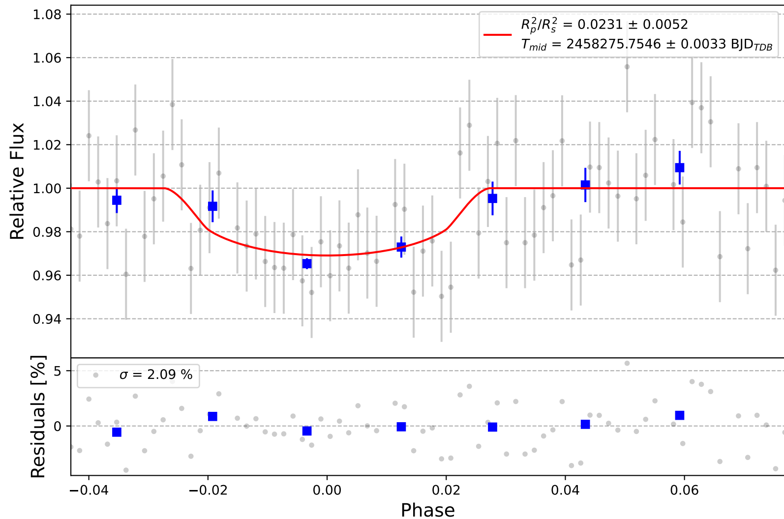
Qatar-2 b
