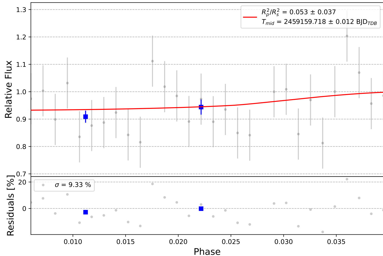
Qatar-4 b
