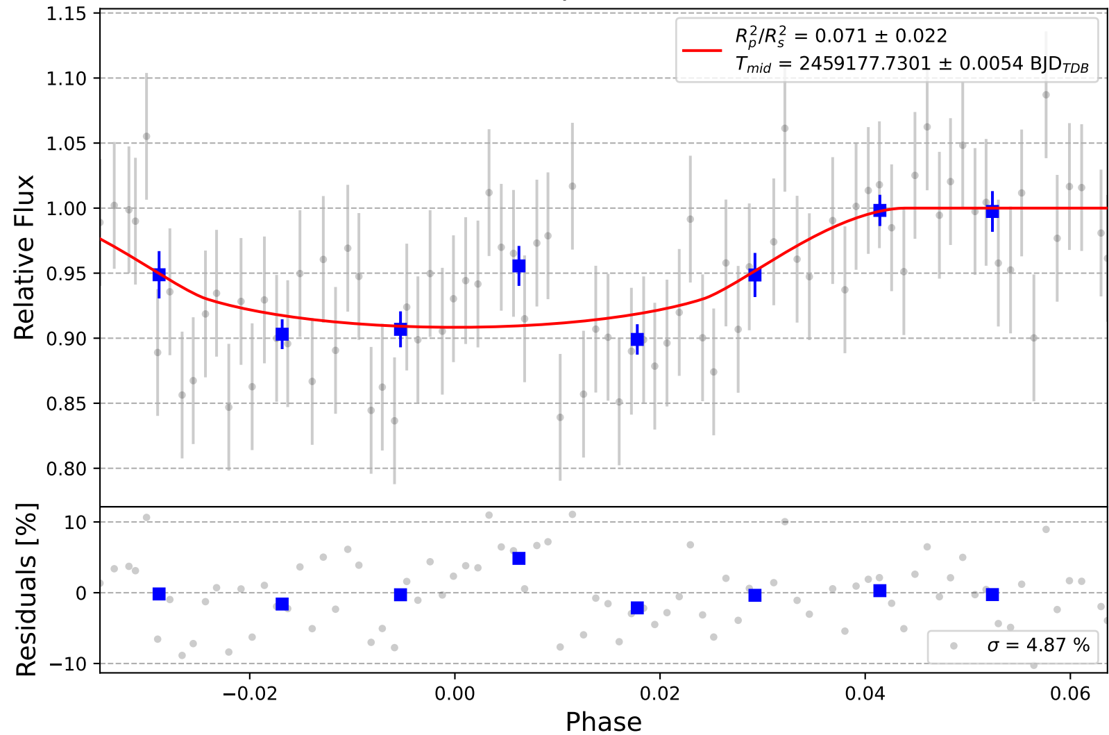
Qatar-4 b
