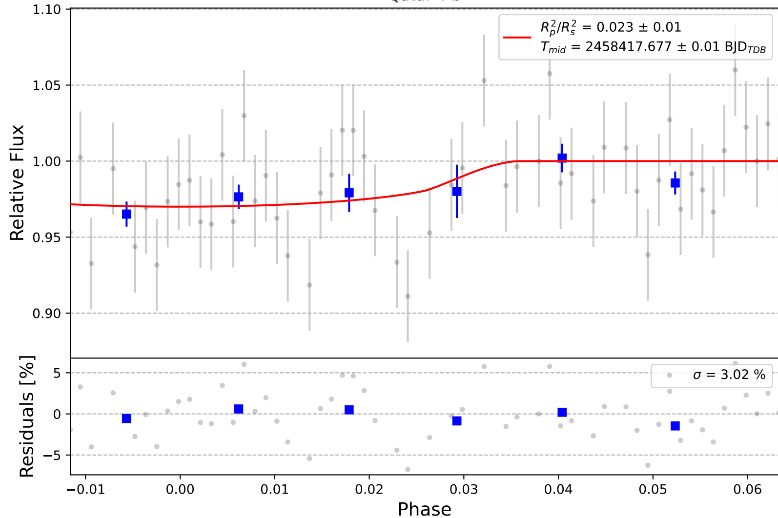
Qatar-4 b
